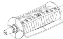
CH Rotor
